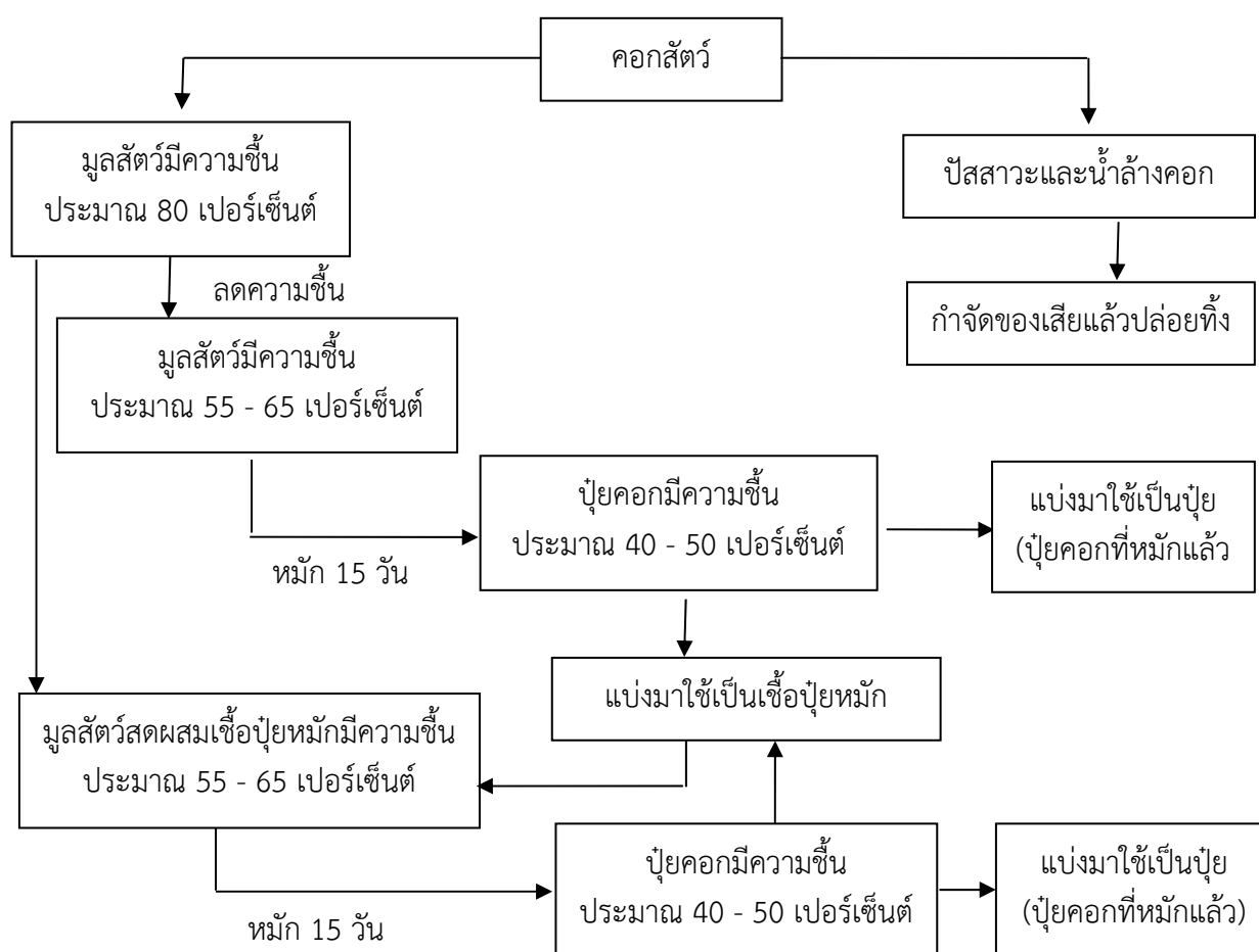
ภาพที่ 4.2 วิธีการหมักมูลสัตว์แบบต่อเนื่อง ที่มา: Matsuzaki (1977)
